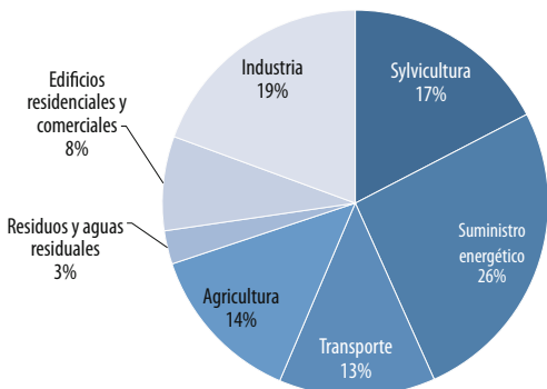
Gráfico 3: Principales contribuidores a las emisiones de gases de efecto invernadero , incluidos el uso de las tierras y el cambio en la cobertura de las tierras (medidos en equivalentes de CO 2 que utilizan un potencial de calentamiento global de 100 años).
