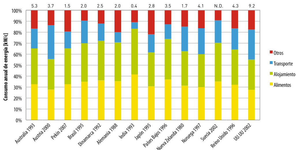
Gráfico 9: Distribución del uso directo e indirecto de energía en los hogares por categorías de consumo, tal y como se identifican en diferentes estudios, y uso total de energía medido en kW per cápita
