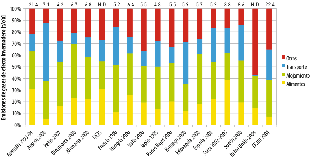
Gráfico 10: Emisiones de CO 2 /gases de efecto invernadero para un conjunto de países, a partir de 22 estudios diferentes
