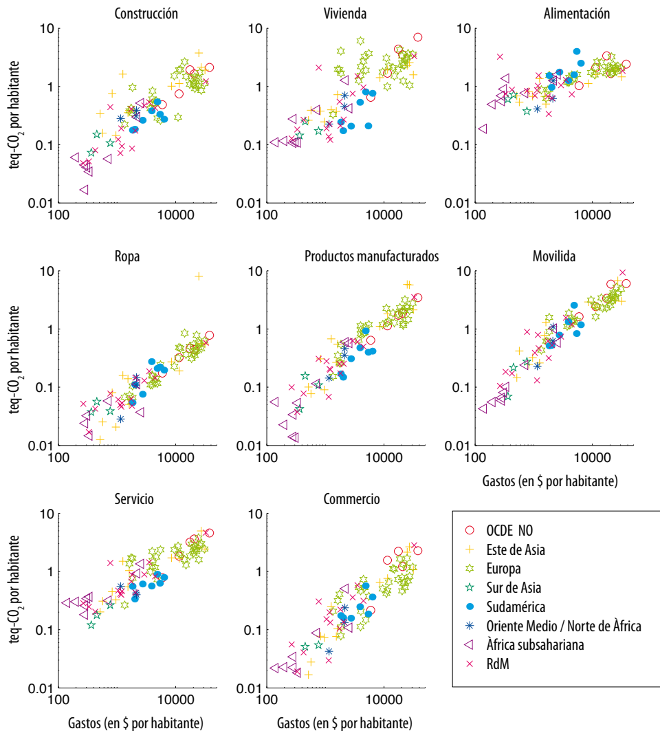
Gráfico 14: Huella de carbono (equivalentes de las toneladas de CO 2 per cápita en 2001) de diferentes categorías de consumo en 87 países/regiones como una función del gasto (dólares per cápita)
