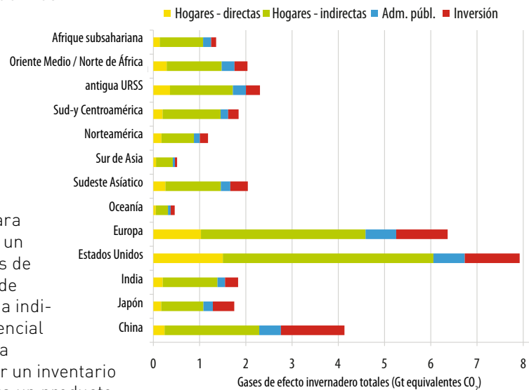
Gráfico 8: Emisiones de gases de efecto invernadero generadas por el consumo de los hogares, el consumo gubernamental y la inversión en diferentes regiones del mundo en 2001.
