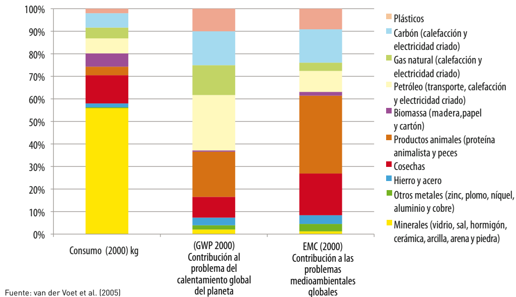
Gráfico 16: Potencial de recalentamiento planetario de los flujos de materiales normalizado y consumo de materiales, ponderada por su impacto sobre el medio ambiente (EMC) para la zona UE
